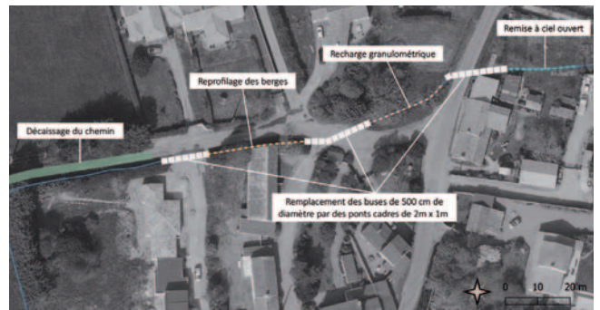
Exemple de pont cadre
